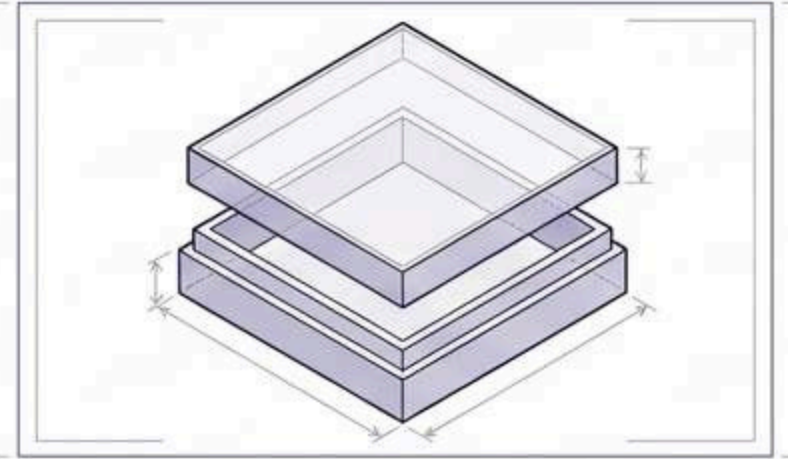
뚜껑·바닥 분리형 상자 (경질 Acrylic 전용)
