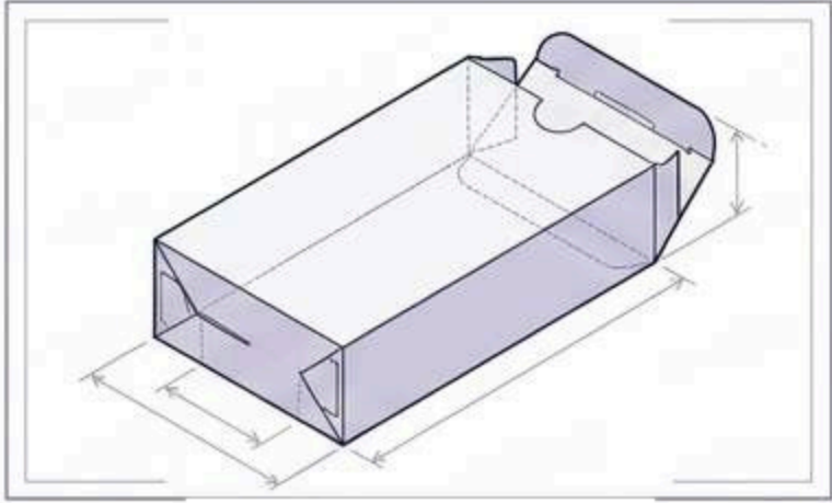
턱엔드 접이식 상자(표준 소매용)
