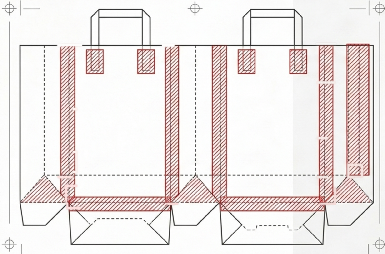
펼친 칼선 도면
